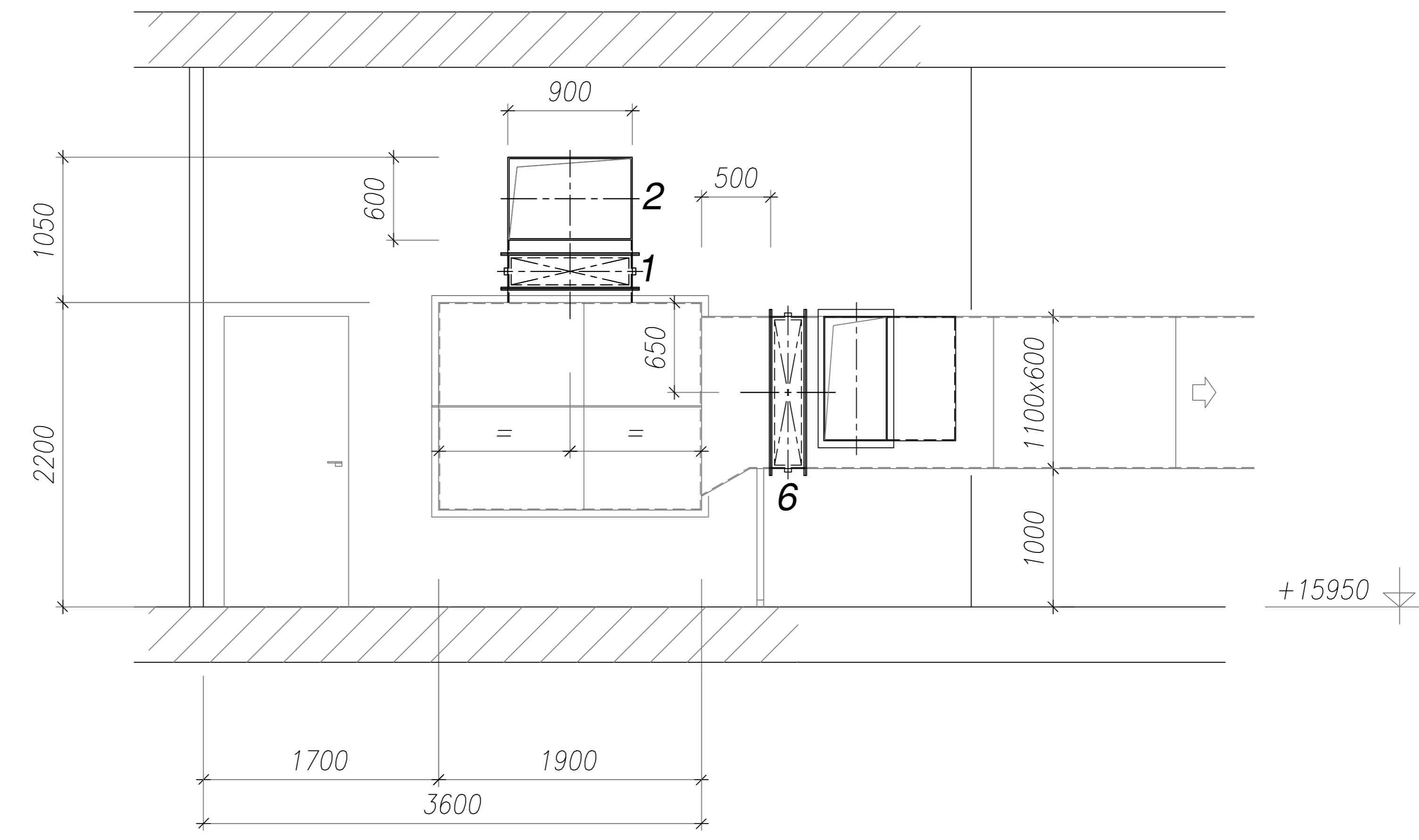
SEZIONE B - B
