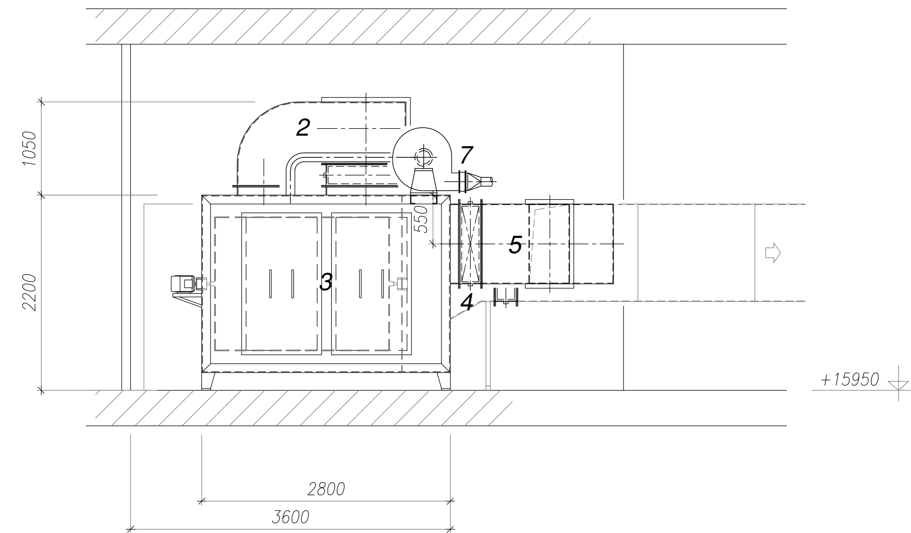
SEZIONE C - C
